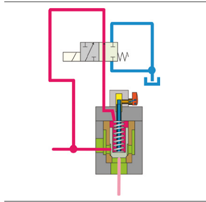
Logikelement mit Wegeventil.
